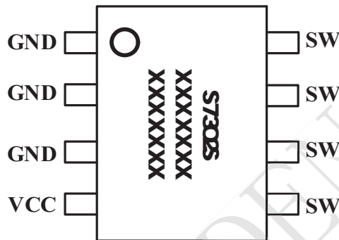
图 2 封装
